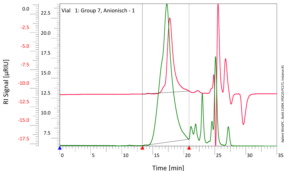
Abb. 6: Die Abbildung zeigt die GPC-chromatografie zu dem erhaltenen Copolymer.
