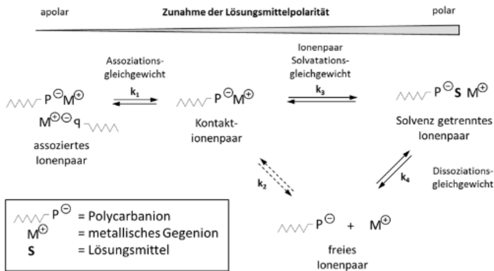
Abb. 1: Die Abbildung zeigt den Einfluss des Lösemittels auf das Gleichgewicht der Ionen im Falle der anionischen Polymerisation. So liegen die Ionen im apolaren Lösemittel als Ionenpaar vor und im polaren Lösemittel als getrennte Ionenpaare.[1]
